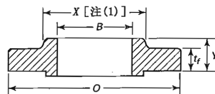
平焊法兰
