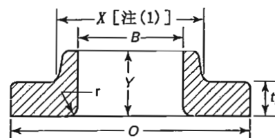
松套法兰
