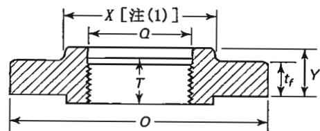
螺纹式法兰
