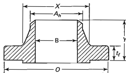
带颈对焊法兰
