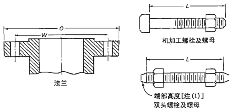
法兰和法兰管件
