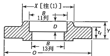
承插焊法兰 (NPS 1/2 至 3)
