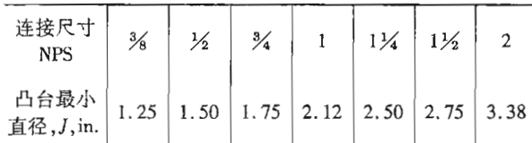
图 II-6 连接用凸台
