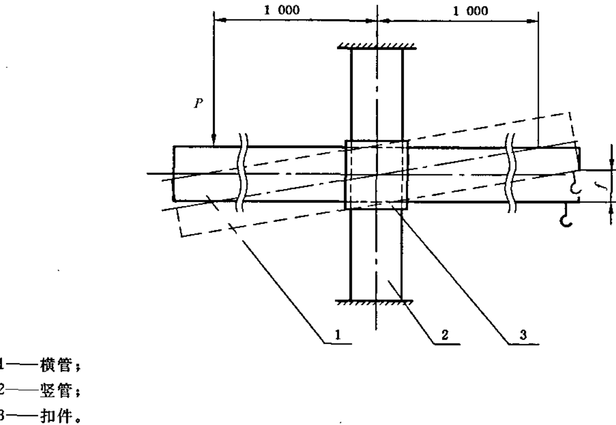
图 4 扣件扭转刚度性能试验示意图
