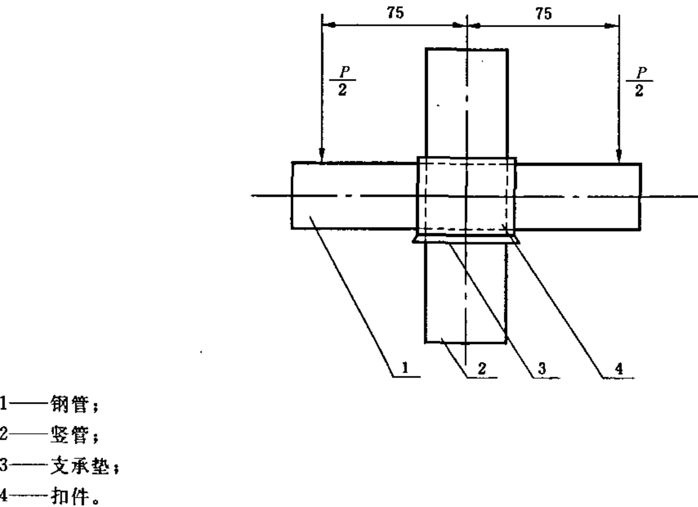
图 3 扣件抗破坏性能试验示意图
