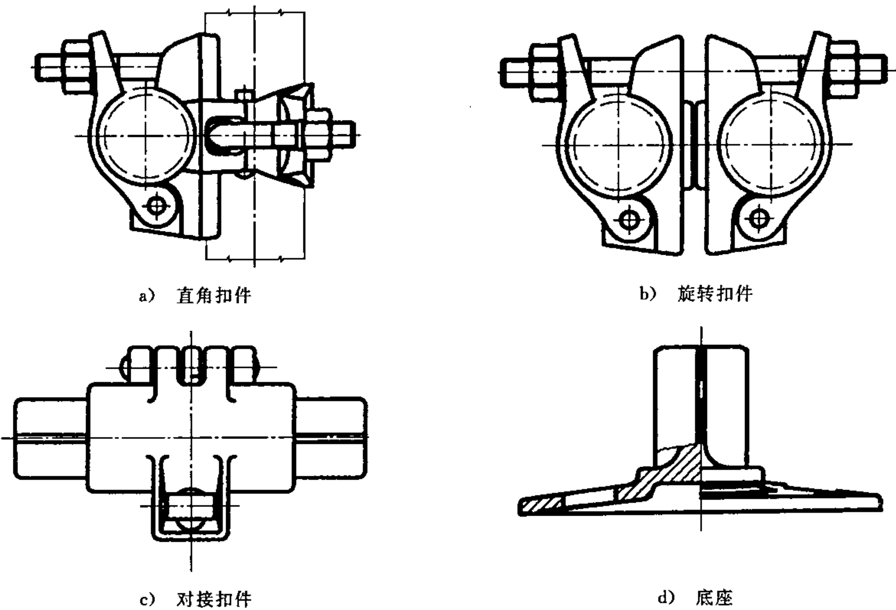
图1 扣件型式示意图
