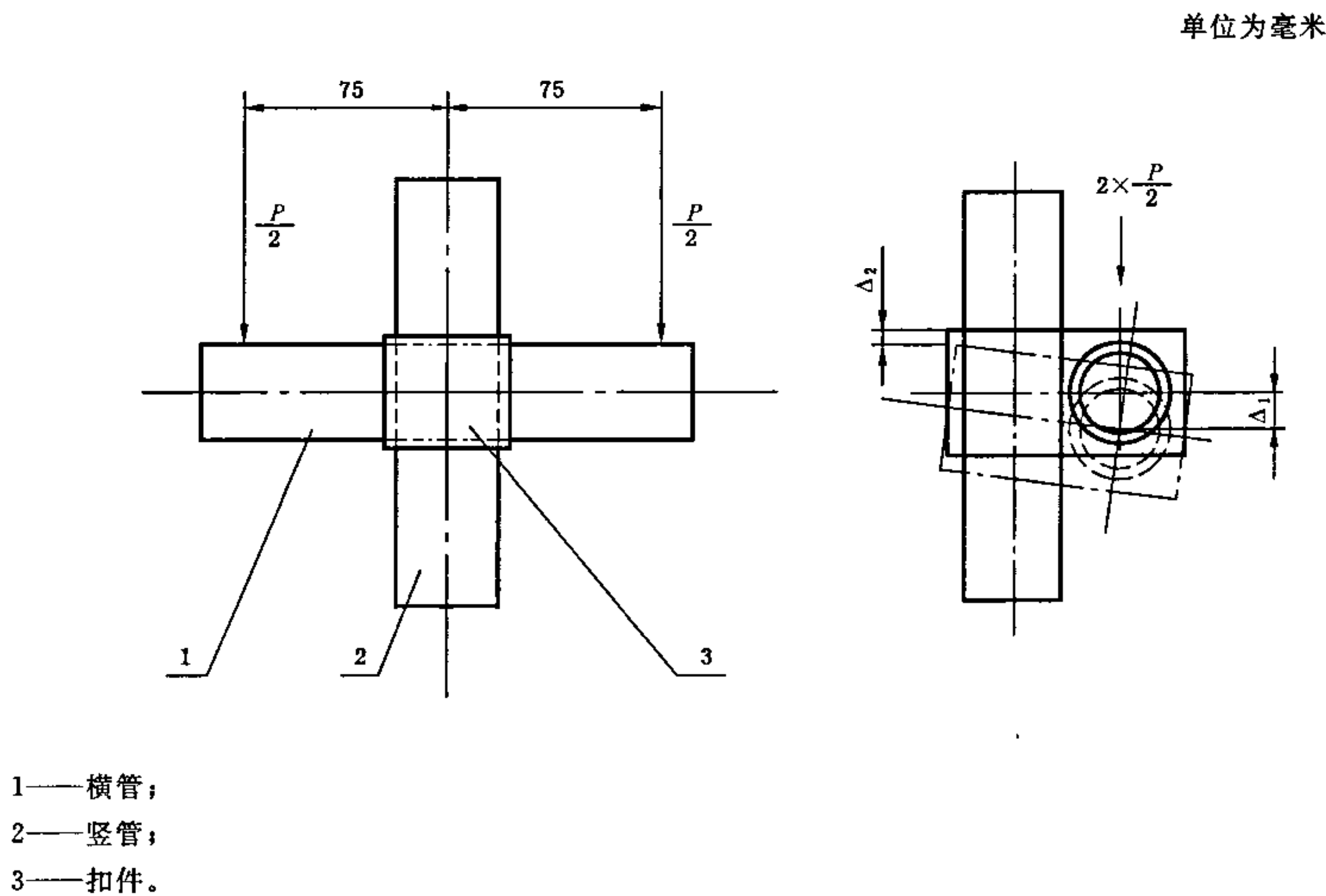
图 2 扣件抗滑性能试验示意图
