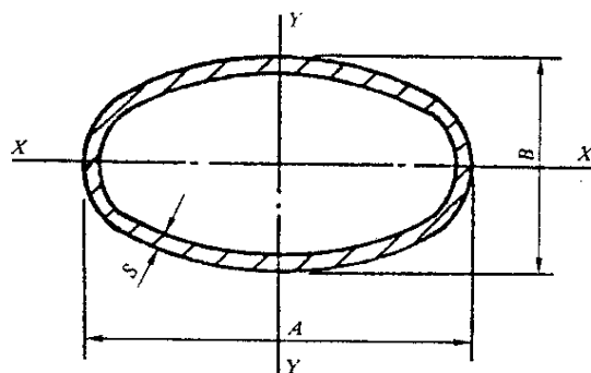
图 A3 D-3 椭圆形钢管
