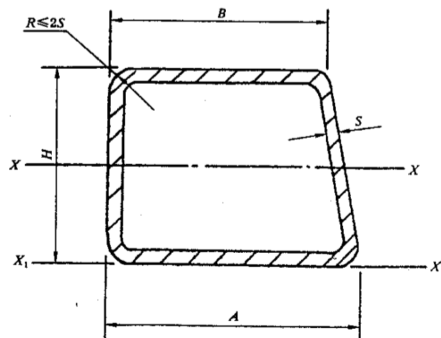
图 A6 D-6 直角梯形钢管
