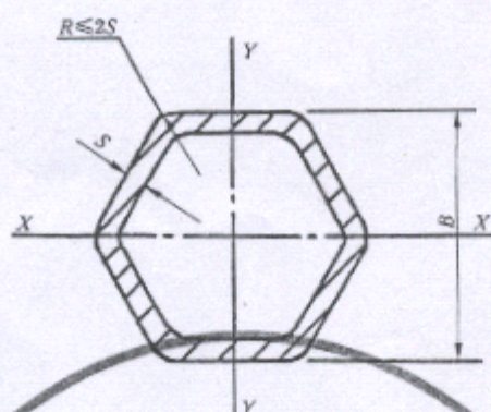
图 A5 D=5 内外六角形钢管 表 A5
