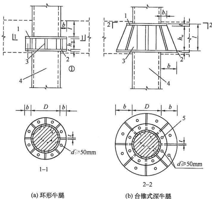
图 7.2.9 环形牛腿构造示意图
