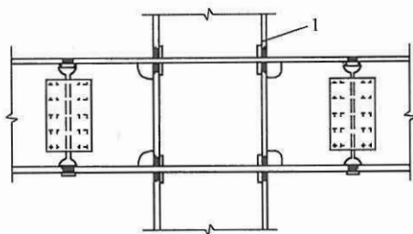
(a) 立面图
