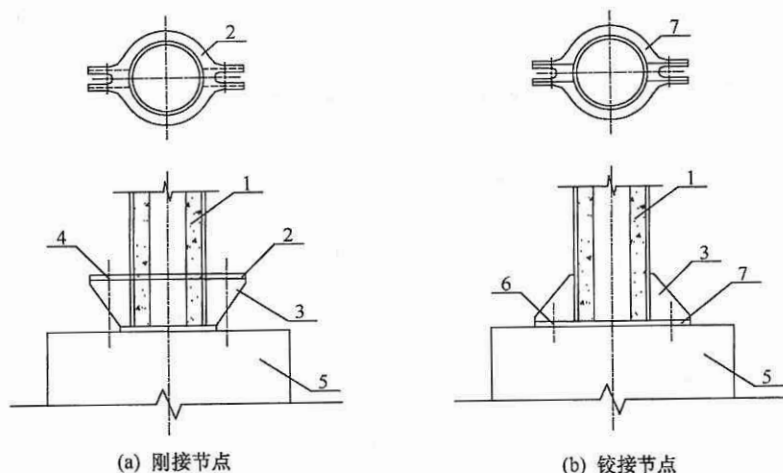
图 7.4.6 锚栓式柱脚
