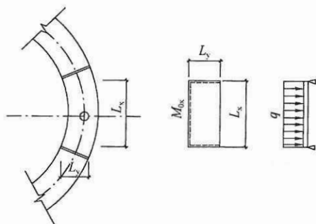
图 7.3.7-2 有加劲板法兰盘受力简图
