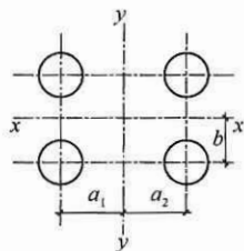
图 5.2.3-3 四肢柱
