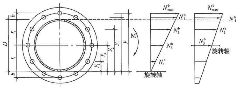
图 7.3.7-1 有劲板法兰螺栓连接
