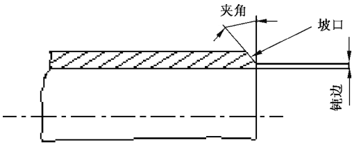
图 2 坡口示意图
