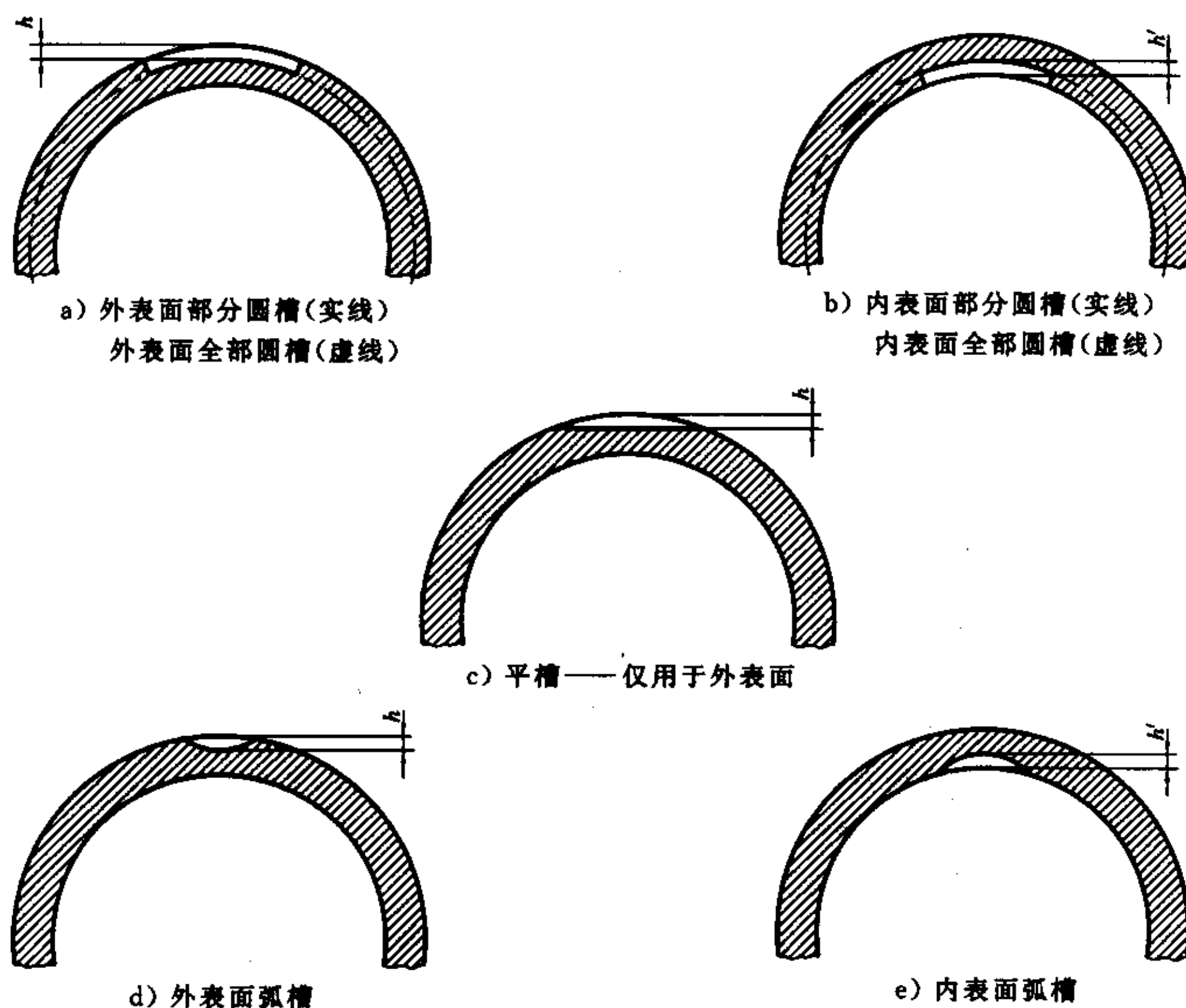
图 4 横槽种类
