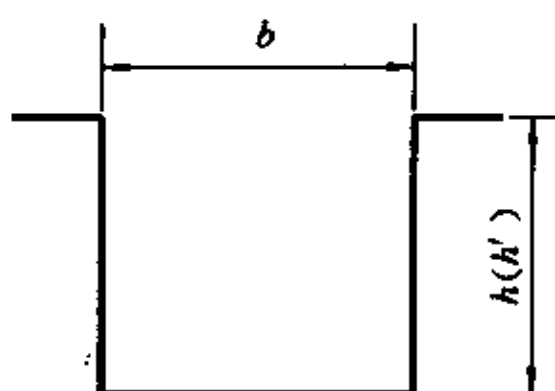
图 3 刻槽
