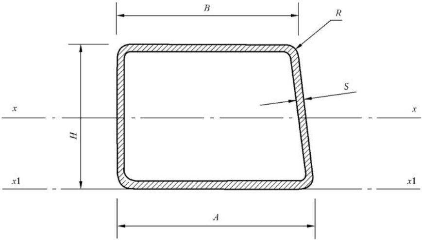
图 A.6 直角梯形钢管(D-6)
