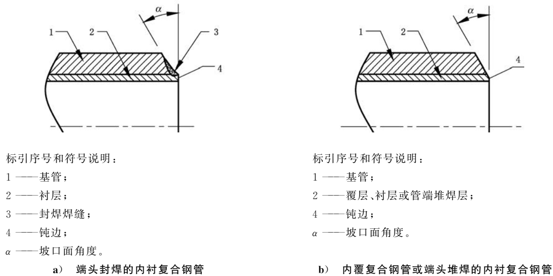
图 2 坡口示意图
