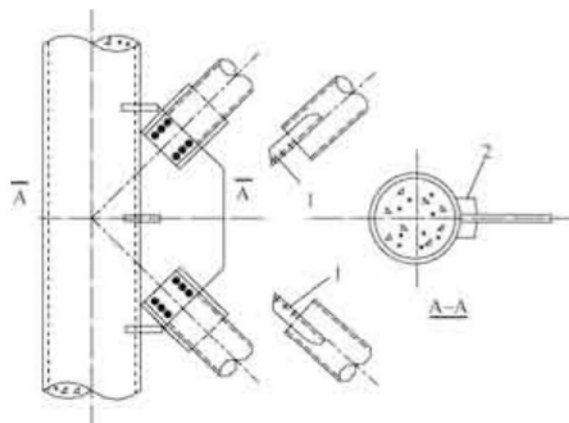
图 8.1.6 节点板连接构造形式 1—插板；2—加劲板
