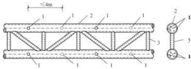
图 9.3.7-1 钢管混凝土桁式混合结构排气孔位置示意 1—排气孔；2—钢管混凝土弦杆；3—腹杆
