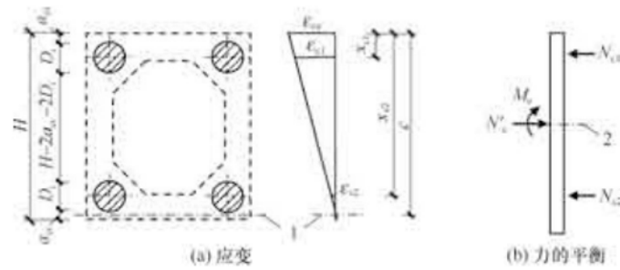
图 7.3.4-2 钢管内混凝土截面的承载力计算示意 [(H-a_{ci}) \leq c \leq H]
