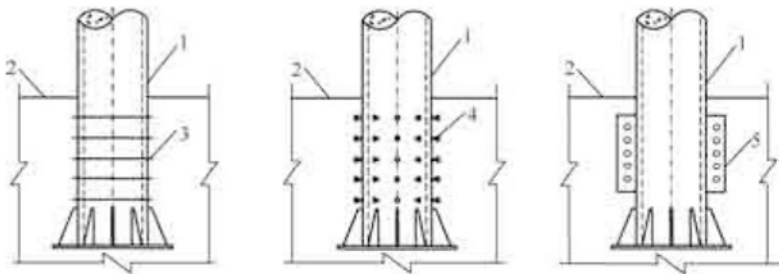
图 8.4.1-2 埋入式连接 1—弦杆；2—基础；3—贴焊钢筋环；4—圆头焊钉；5—开孔板连接件
