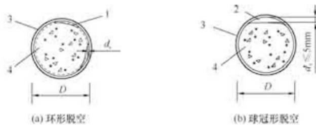
图 10.3.10 混凝土脱空尺寸示意
