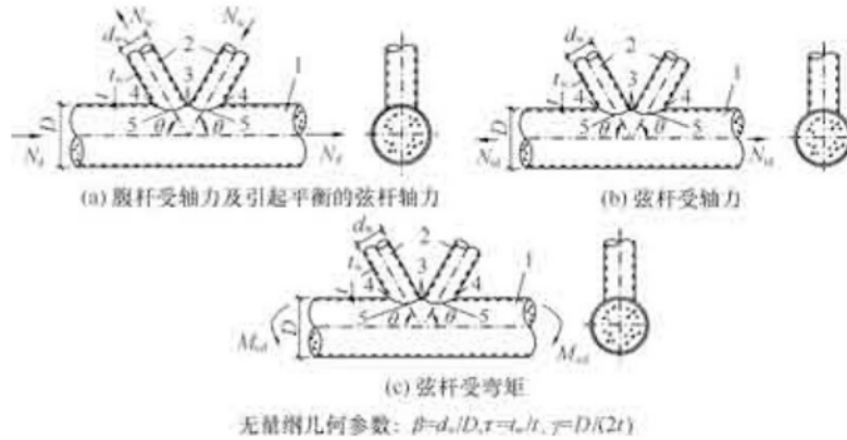
图 D.0.2 K 形间隙节点受力形式示意
