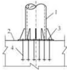
图 8.4.1-1 端承式连接 1—弦杆；2—基础；3—承压板；4—锚栓
