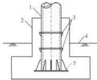
图 8.4.1-3 外包式连接
