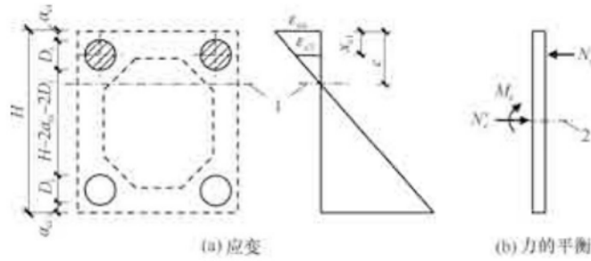
图 7.3.4-4 钢管内混凝土截面的承载力计算示意
