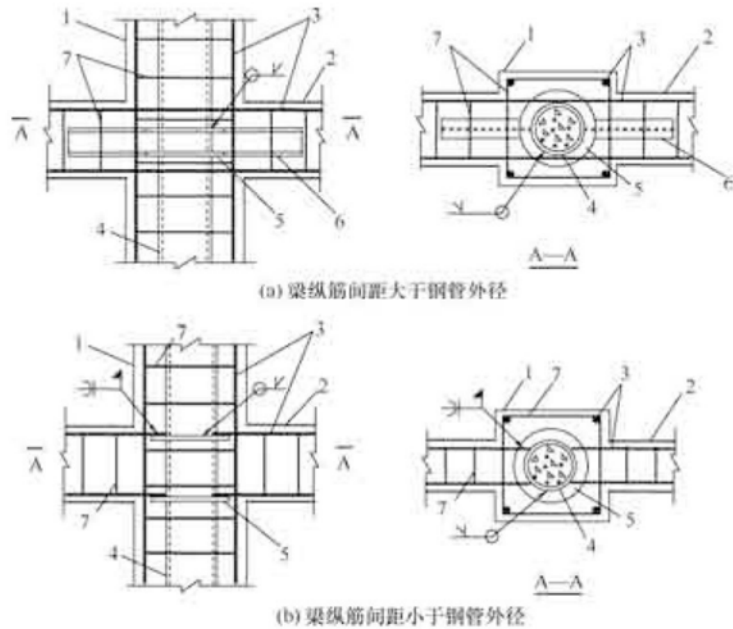
图 8.3.2 柱与钢筋混凝土梁连接节点
