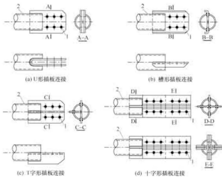
图 8.1.5 不同类型的腹杆端部插板连接构造形式 1—螺栓；2—腹杆
