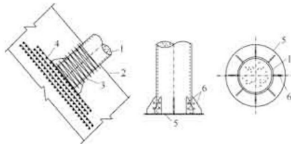
图 8.4.3 曲线形结构与基础的连接构造
