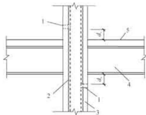
图 9.3.7-2 钢管混凝土加劲混合结构排气孔位置示意 1—排气孔；2—内置钢管混凝土；3—外包混凝土；4—钢梁；5—楼板
