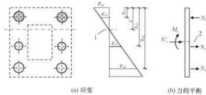
图 7.4.4 钢管截面的承载力计算示意
