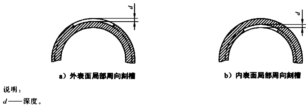
图 2 典型的横向刻槽
