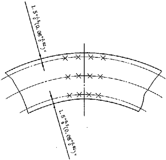
a) SMLS 钢管
