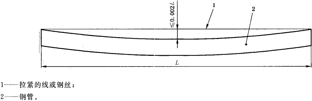
图 1 全长直度测量
