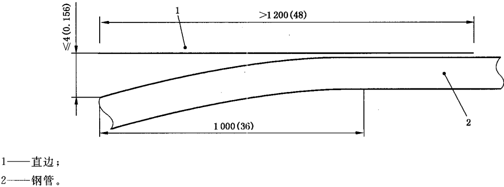
图 2 端部直度测量
