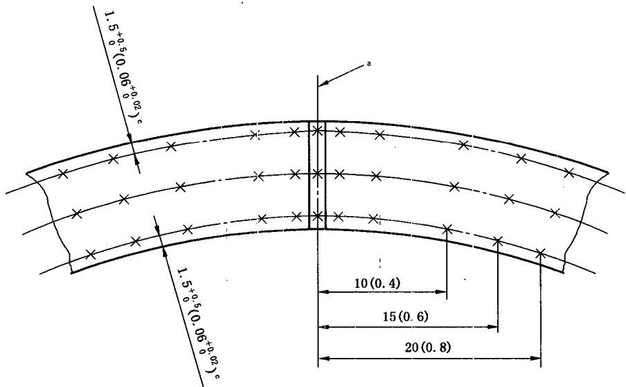
c) HFW 钢管
