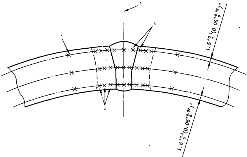
b) SAW 钢管
