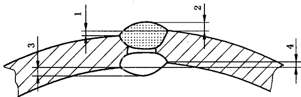
b) SAW 钢管错边和焊缝高度
