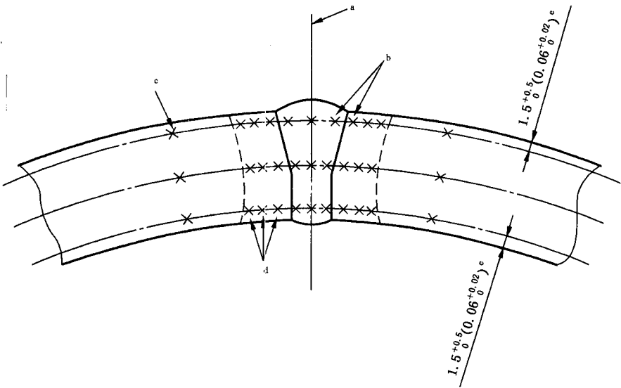
b) SAW 钢管
