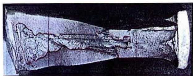
c) 第Ⅲ类异常断口
