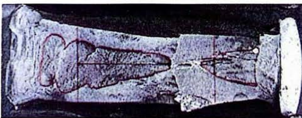
d) 第Ⅳ类异常断口
