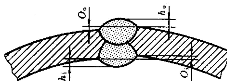
b) 钢板或钢带边缘的径向错边及焊道高度 (SAW 和 COW 钢管)
