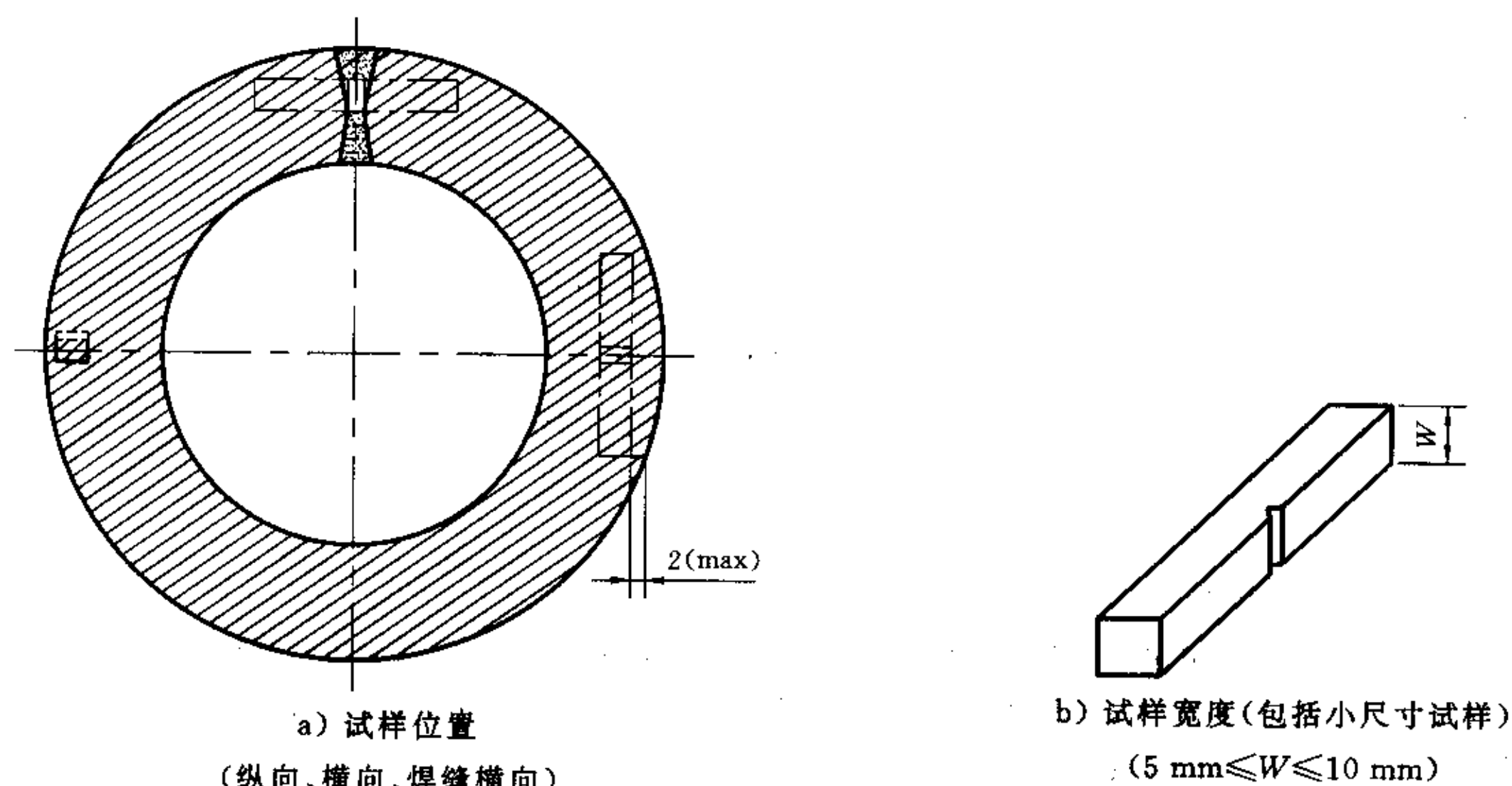
图 5 冲击试样位置和宽度
